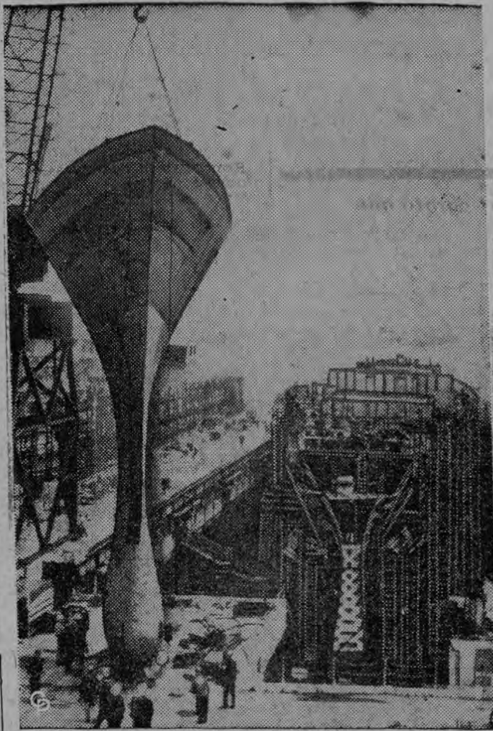
PROA PARA CRUCERO NUCLEAR: Con un peso de 70 toneladas, la proa de 56 pies de alto, del crucero movido por energía nuclear USS Long Beach, es colocado en su lugar para ser soldado (derecha). El navío está bajo construcción en los astilleros de la Bethlehem Steel Company de Quincy, Mass. Será bautizado en junio 20
